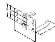
Für 35 mm Schienenmontage
